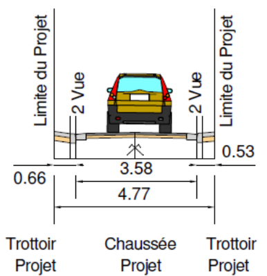
Profil AA' Projet
