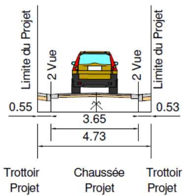
Profil BB' Projet
