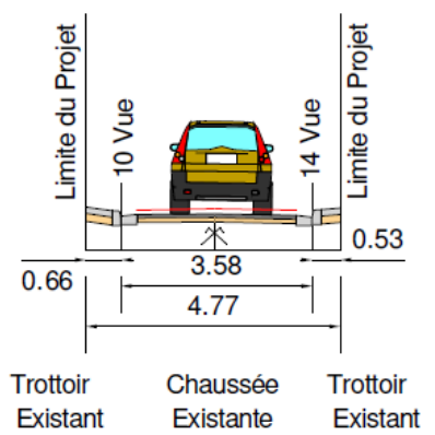
Profil AA' Existant
