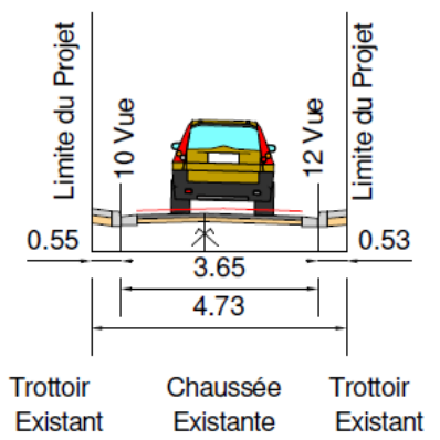
Profil BB' Existant
